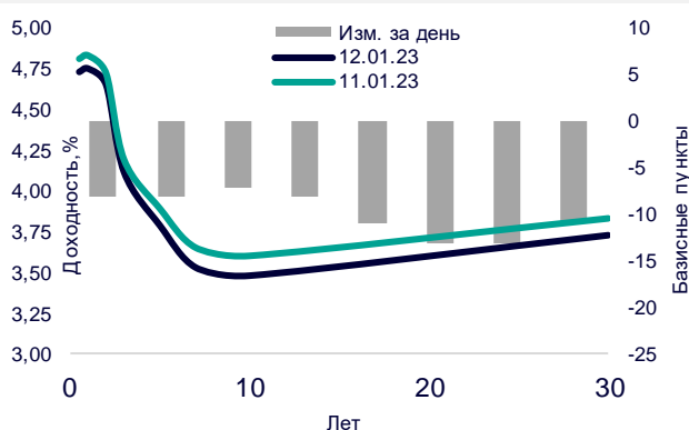
Кривая ОФЗ
