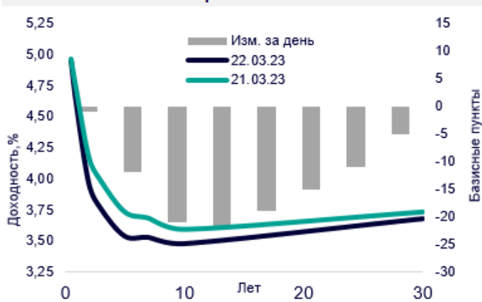
Кривая ОФЗ
