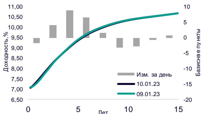
Кривая ОФЗ
