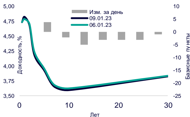
Кривая ОФЗ
